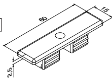
Bottom
